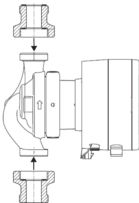
Рис. 71 Пример резьбовых переходников
