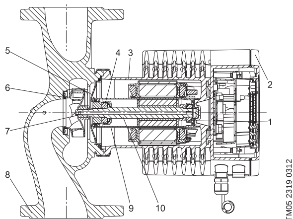
Рис. 46 Исполнение с фланцем
