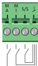
Рис. 54 Цифровой вход в блоке управления
