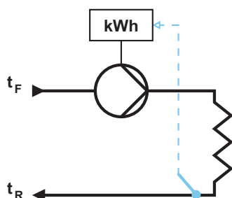
Рис. 37 Насос MAGNA3 со встроенным счетчиком тепловой энергии.
