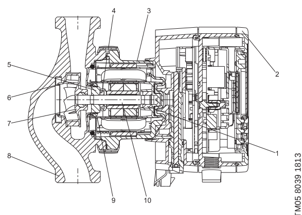
Рис. 47 Исполнение с резьбой
