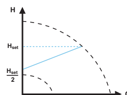
Пропорциональное давление
