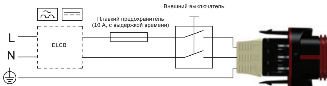
Рис. 50 Пример подключения со штекером ALPHA, 1 x 230 В ± 10 %, 50/60 Гц, защитное заземление
