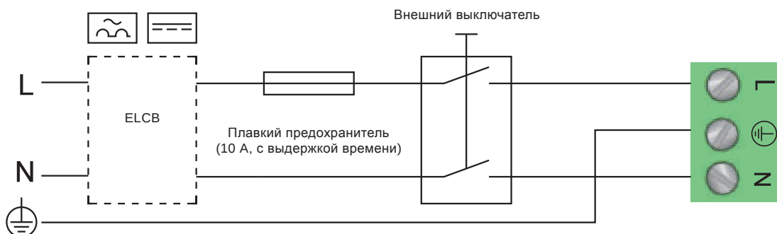
Рис. 52 Пример типового подключения, 1 х 230 В ± 10 %, 50/60 Гц
