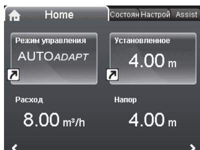
Рис. 35 Меню "Home"
