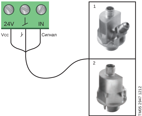
Рис. 58 Примеры внешних датчиков
