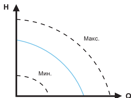
Рис. 13 Максимальная и минимальная характеристики
