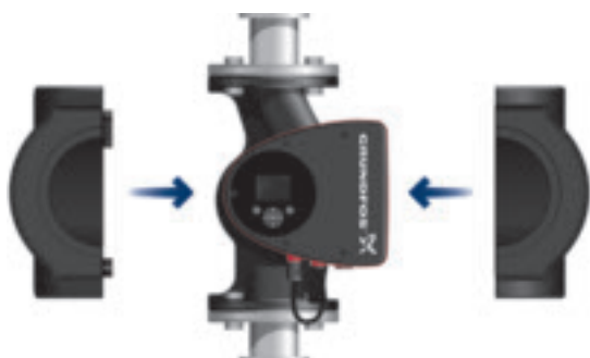
Рис. 63 Установка теплоизоляционного кожуха на насос MAGNA3
