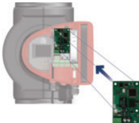
Рис. 65 Расположение модуля CIM
