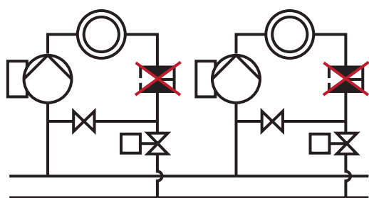
Рис. 15 Меньшее количество необходимых дроссельных клапанов насоса
