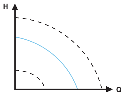
Рис. 25 Режим эксплуатации по постоянной характеристике
